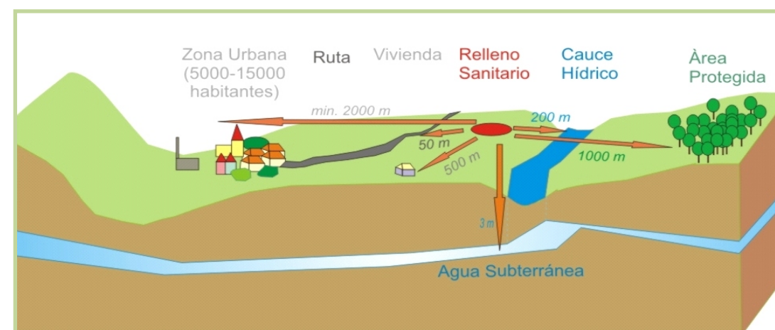
Fig.n°38: Implantación correcta para un vertedero. Fuente: ORDAZUR/SEAM
