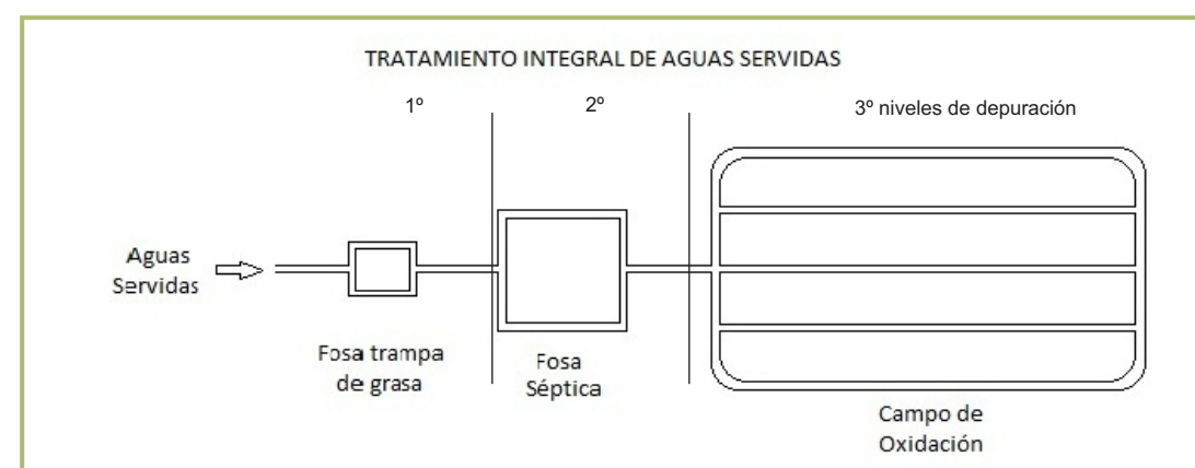
Fig. n° 37: Alternativa de tratamiento doméstico de aguas servidas. Fuente: http://www.autosuficiencia.com.ar . Gráfico: elaboración propia
